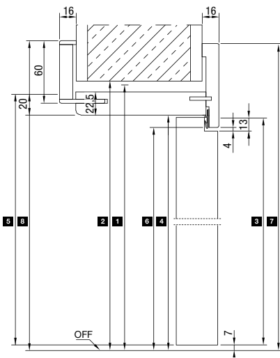
Verticale doorsnede
