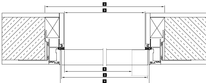
Horizontale doorsnede met reverse openend deurblad
