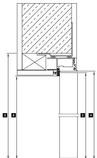
Verticale doorsnede met stomp deurblad
