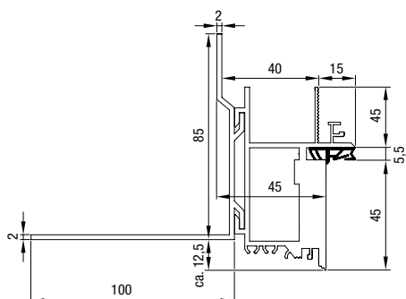
Maten Zeroline-kozijn
